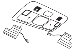
③ LEDの取り付け
