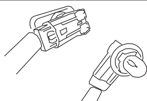
②ナンバーランプソケットの取り外し
