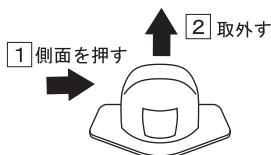
① ランプユニットの取外し
