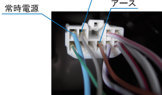
ウェルカム配線 ドアオープン時にマイナスになる配線
