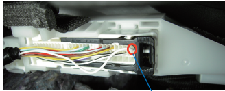
ウェルカム配線 ドアオープン時にマイナスになる配線
